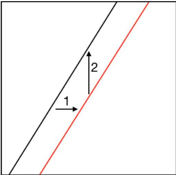
그림1 로그 축척으로 그리면 거듭제곱 함수는 곧은 직선의 꼴이 된다. 가로축 방향으로 평행이동(1번 화살표)하고 나서 다음에 세로축 방향으로 적당한 평행이동 (2번 화살표)을 하면 원래의 직선에 겹쳐지게 할 수 있다. 거듭제곱 함수만 이렇게 할 수 있으니, 거듭제곱함수만 척도가 없다. 직선이 아닌 곡선을 아무거나 그리고는 위의 방법으로 다시 겹쳐지게 만들 수 있는지 살펴보라.
