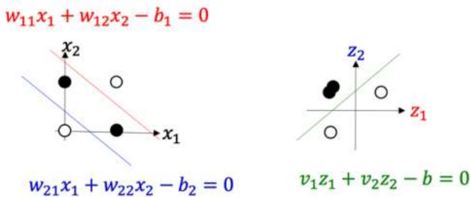
그림6 배타적 논리합을 해결한 숨은층 / 조정호
