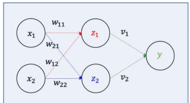
그림6 배타적 논리합을 해결한 숨은층 / 조정호
