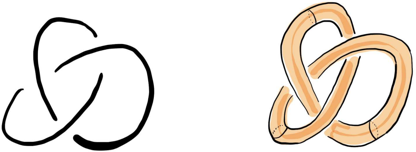
그림2 매듭 K 와 S^1 \times B^2 의 매장 \nu(K) 박정환
