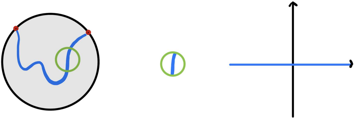
그림1 위상적 단면 매듭 K 와 B^4 에 국소 평탄하게 매장된 B^2
