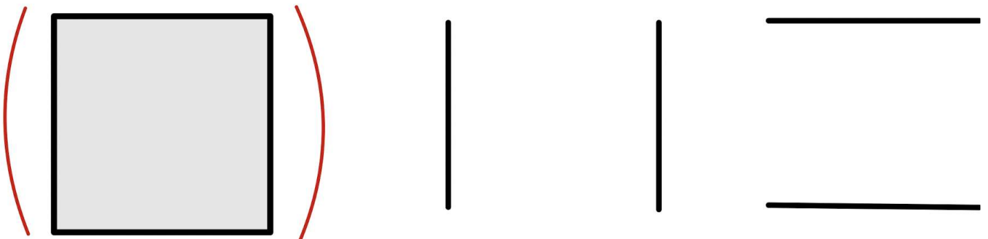
그림3 매듭 K 의 자취 X(K) / 박정환
